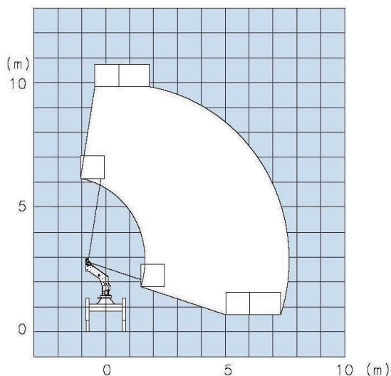
作業半径図
